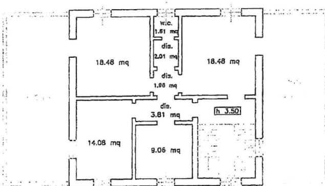
Strada Frassolo PIANO PRIMO
