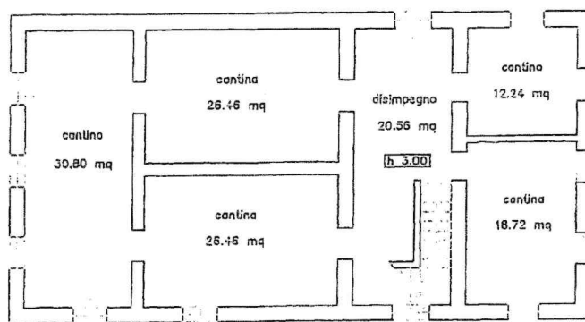
Strada Frassolo PIANO SEMINTERRATO
