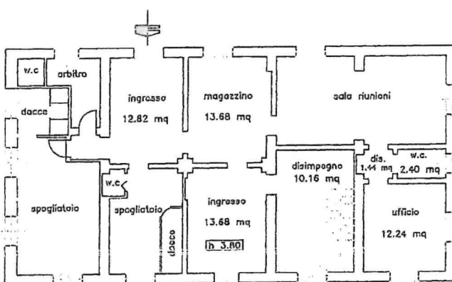
Strada Frassolo PIANO TERRENO
